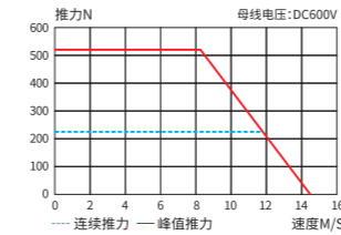
CFS075B滑台380V推力图
